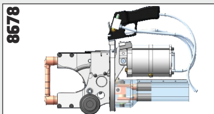
Pinza pneumatica raffreddata ad acqua. Bracci standard e grande apertura.
