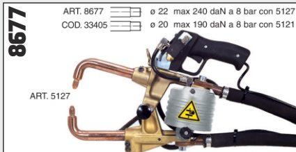
Pinza pneumatica raffreddata ad acqua. Bracci standard e grande apertura art. 5127+5137.
