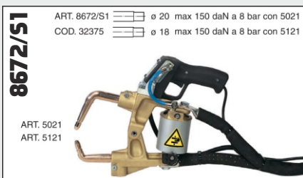
Pinza pneumatica raffreddata ad aria e ad acqua. Bracci standard e grande apertura art. 5001+5085 e art. 5121+5185.
