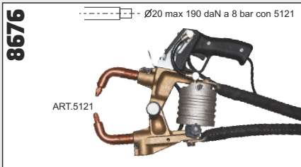
Pinza pneumatica raffreddata ad aria e ad acqua. Bracci standard e grande apertura art. 5001+5085 e art. 5121+5185.
