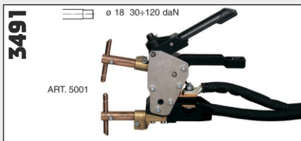
Pinza manuale raffreddata ad aria. Bracci standard e grande apertura art. 5001+5085.
