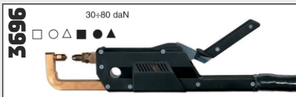
Pinza manuale tipo «C» raffreddamento ad aria. Ingombro ridotto. Lunghezza cavi 1600 mm.
